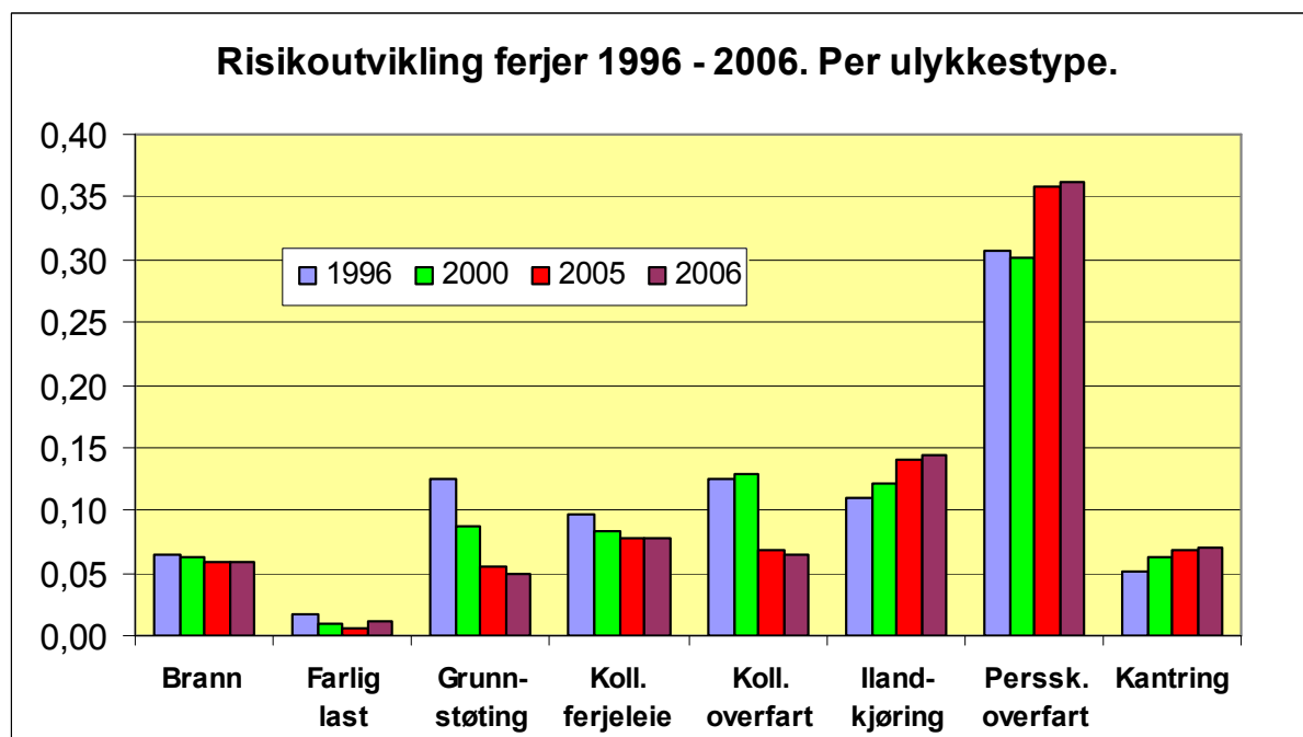
Figur 1 Risiko(beregnet antall omkomne per år) for årene 1996-2006 fordelt på ulykkestyper
